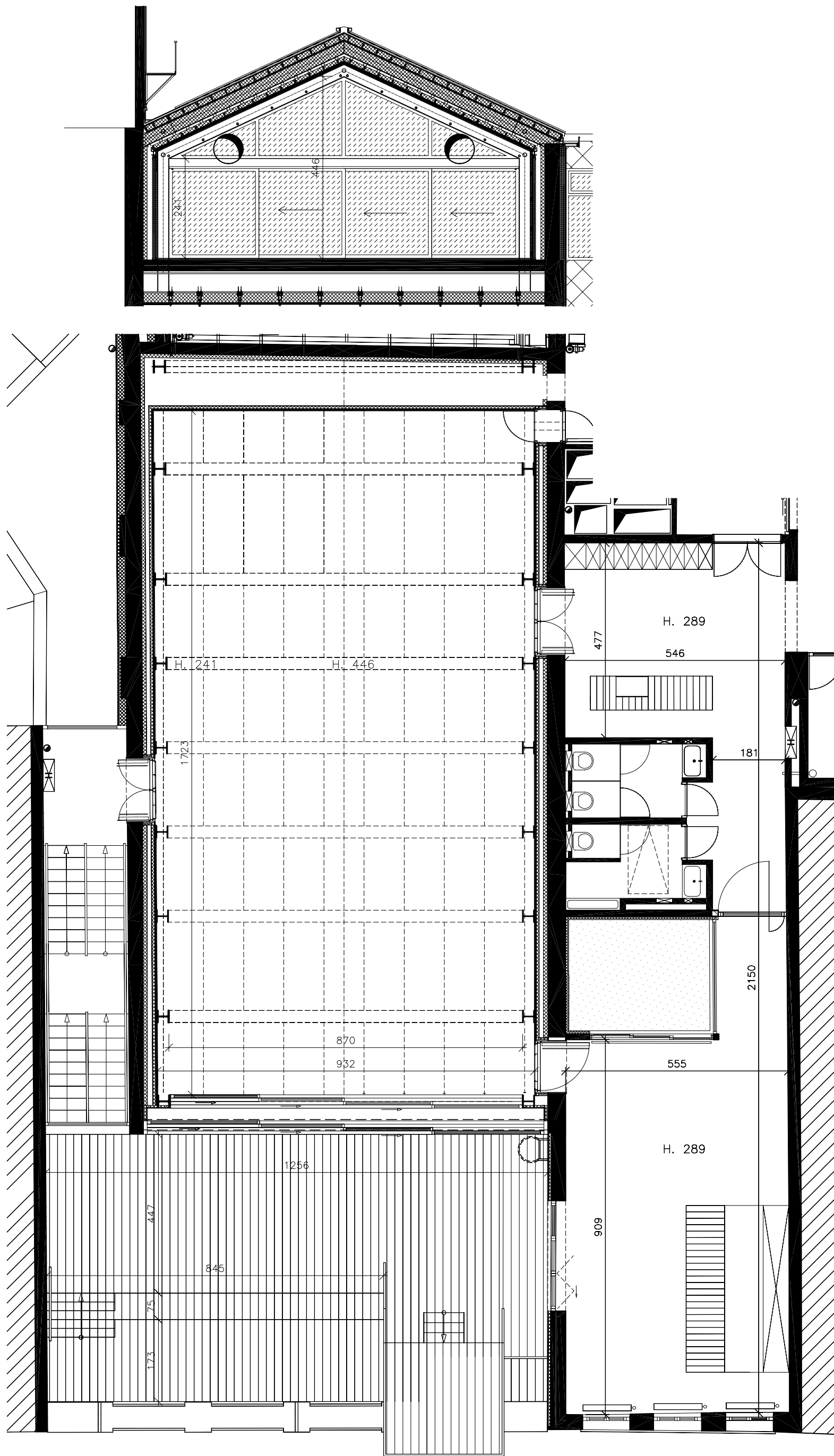
Beursschouwburg Brussel 5de V - zolderzaal / buitenterras + foyer plan + snede 1/100
