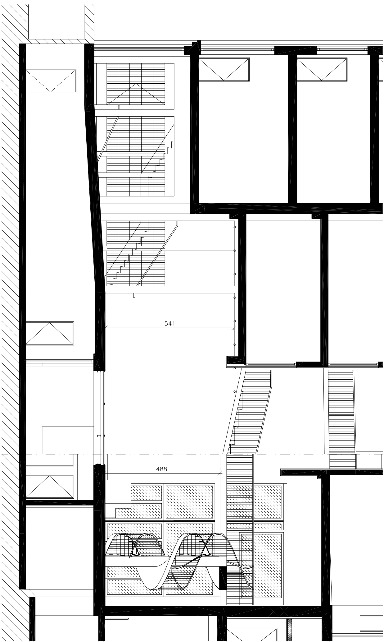
Beursschouwburg Brussel GELIJKVLOERS - centrale hal snede BB 1/100
