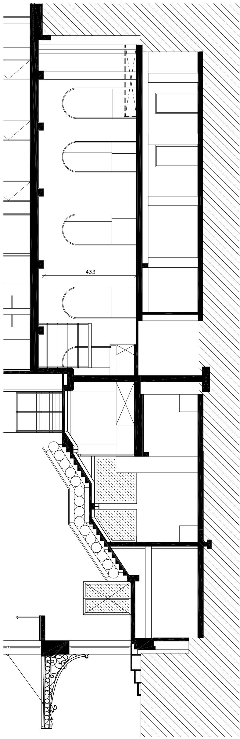
Beursschouwburg Brussel GELIJKVLOERS - Centrale Hal snede 1/100
