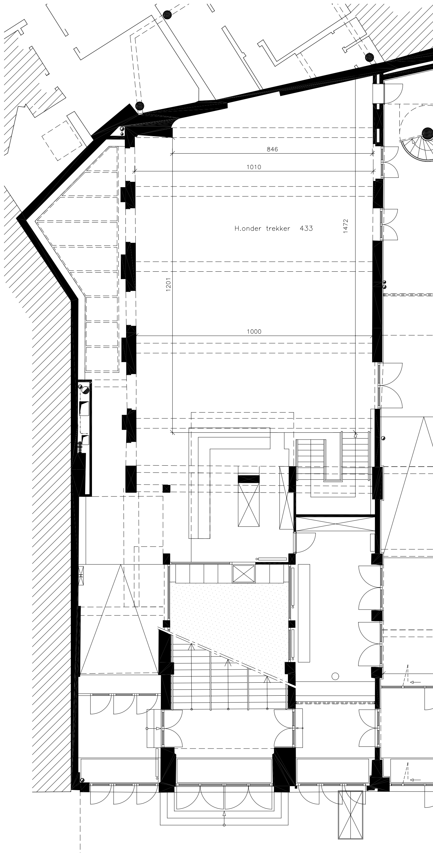
Beursschouwburg Brussel GELIJKVLOERS - inkom + beurscafé plan 1/100
