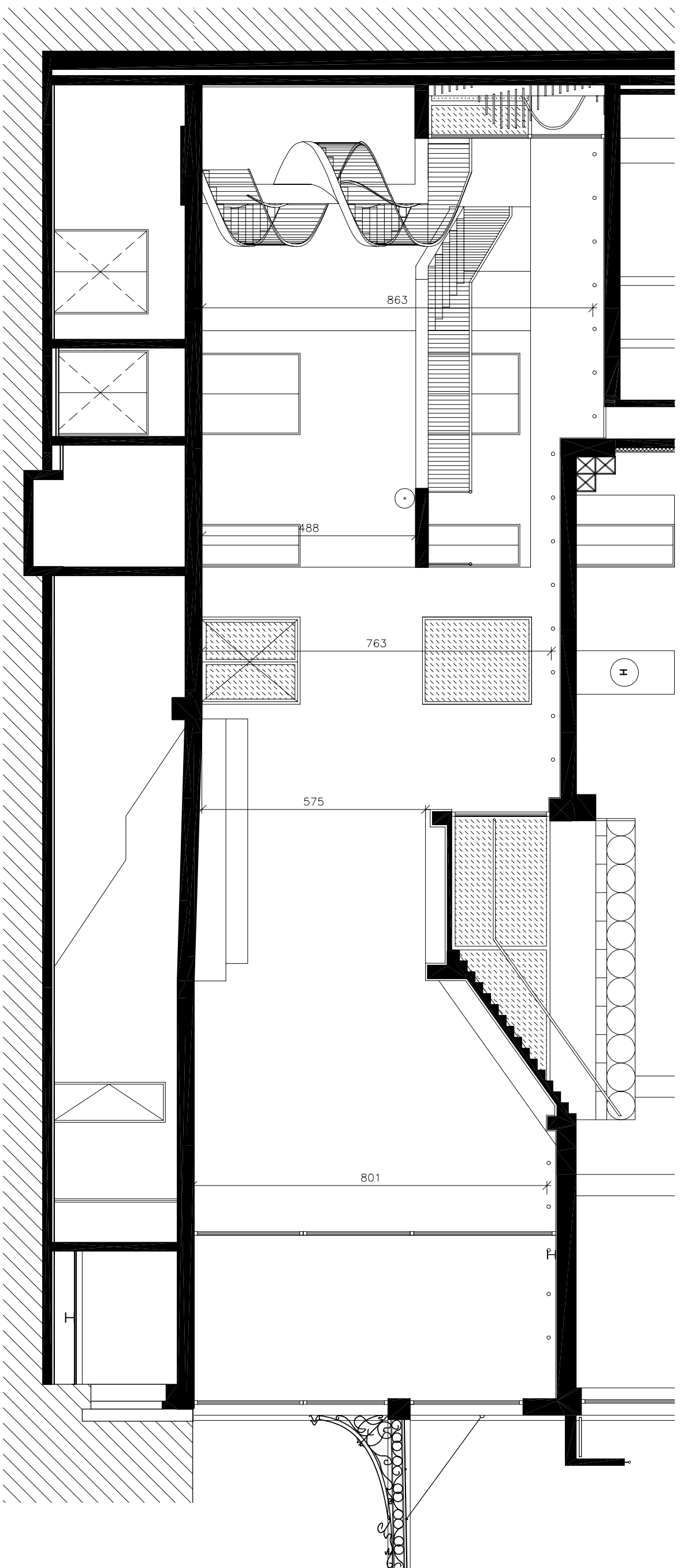
Beursschouwburg Brussel GELIJKVLOERS - centrale hal sneede AA 1/100
